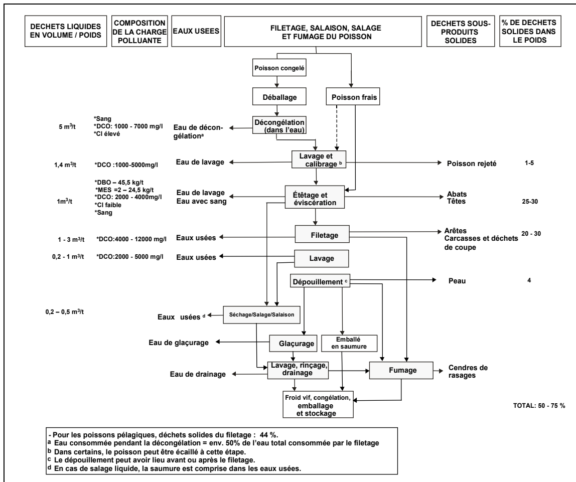
Figure 3.26 : Niveaux de consommation et d'émission enregistrés au cours des séquences processuelles de découpage en filets et de conservation du poisson [134, AWARENET, 2002]
