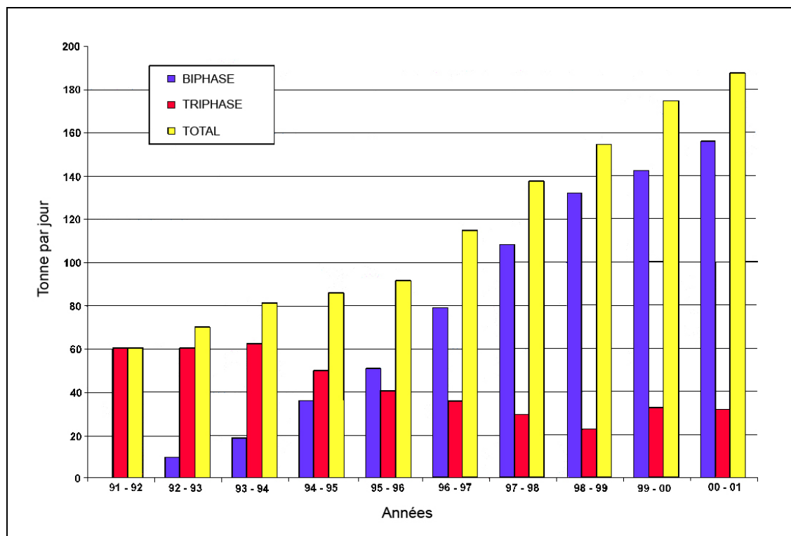
Figure 4.94 : Procédés d'extraction de l'huile d'olive bi-phase et tri-phase [86, Junta de Andalucía and Agencia de Medio Ambiente, 1994]
