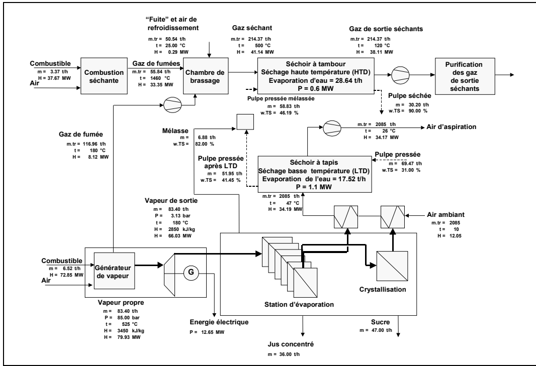
Figure 4.112 : Procédé de déshydratation bi-phase de la pulpe
