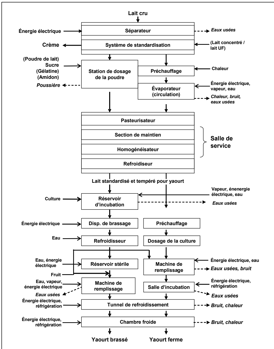
Figure 2.16 : Production de yaourts [9, Verband der Deutschen Milchwirtschaft (German Dairy Association), 1999]
