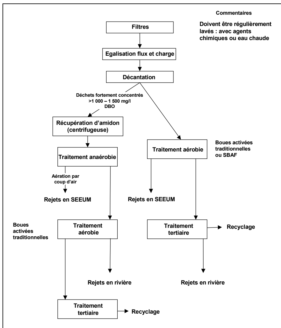
Figure 4.82 : Schéma de principe type du traitement des eaux usées applicable au secteur des fruits et légumes [13, Environment Agency of England and Wales, 2000]
