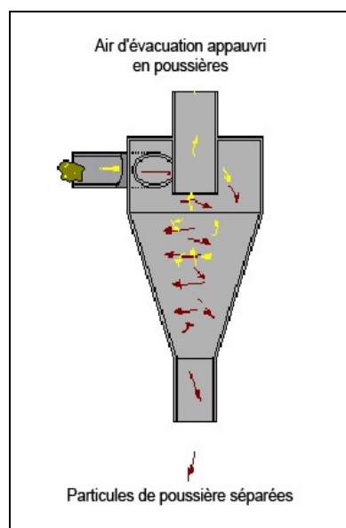
Figure 4.64 : Schéma de principe du cyclone
